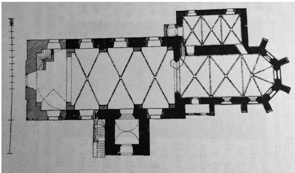
Půdorys kostela. Plná černá barva značí dobu románskou – přechodní, křížováním dobu gotickou, husté čárkování dobu renesanční a barokní, řidší čárkování dobu 19. století (zdroj: Místopis Řečice Kardašovy II.)
